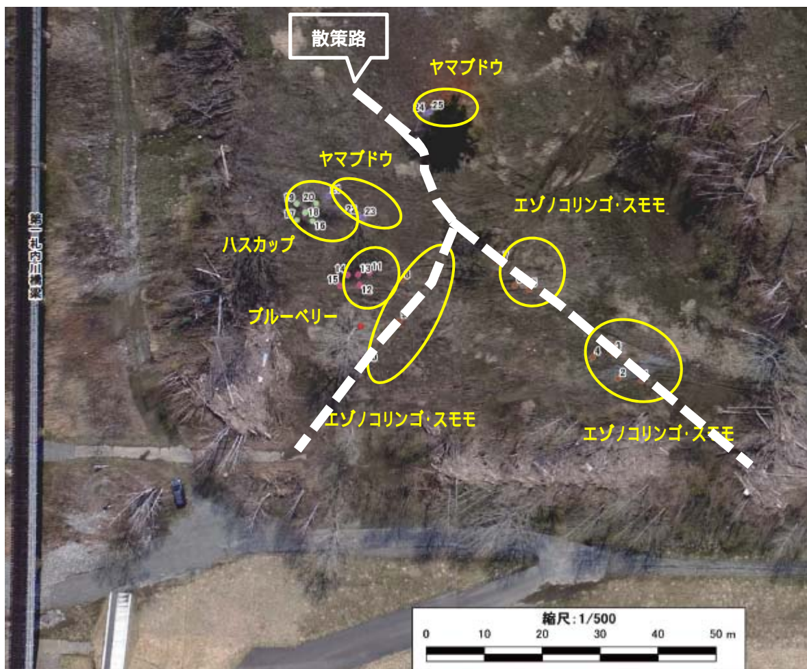
光南地区 水辺の楽校 植樹平面図
