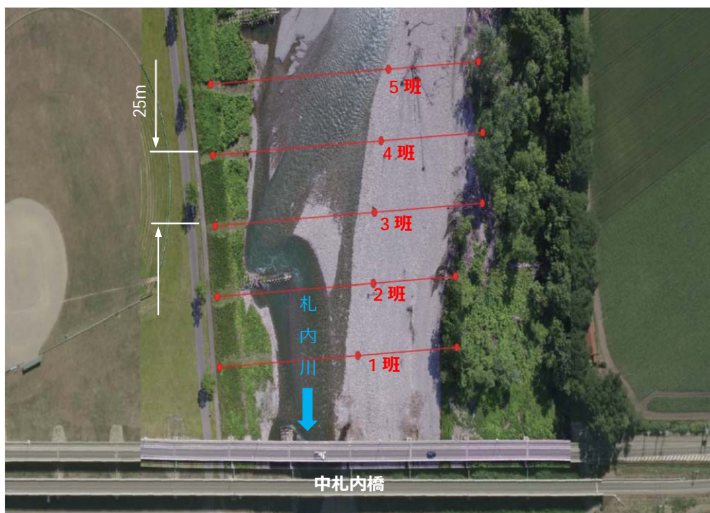
横断測量箇所航空写真
